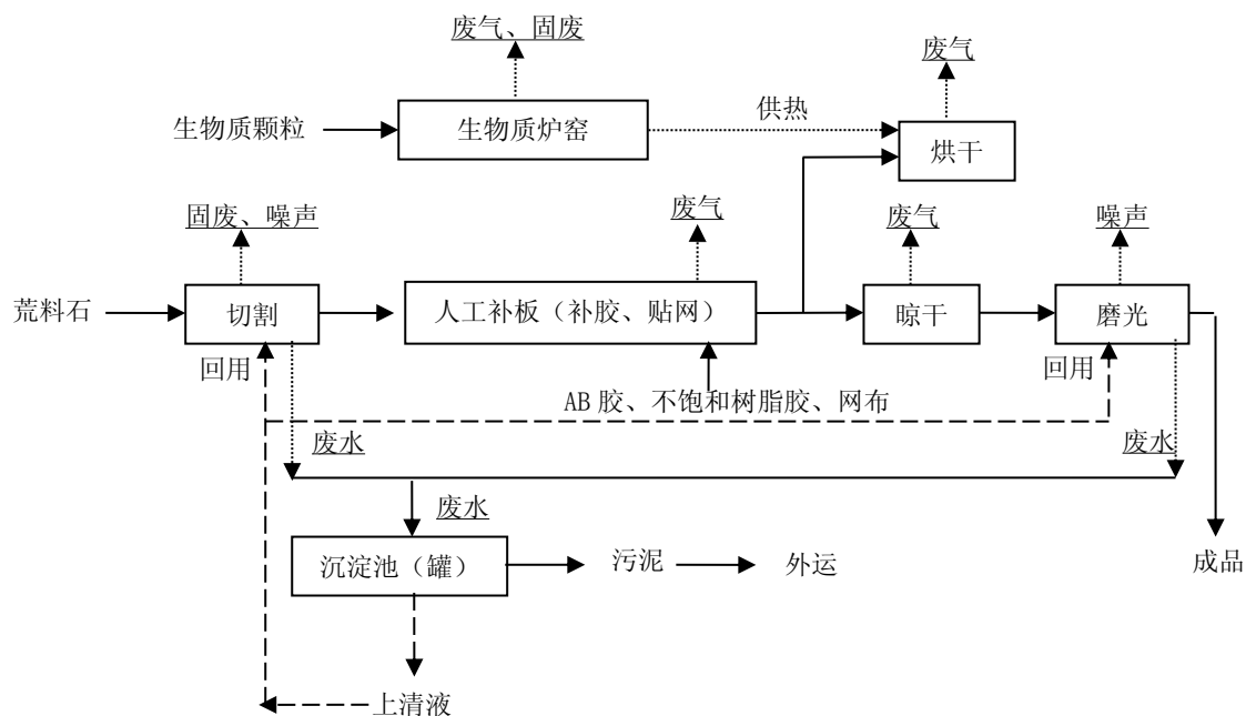
图 3-2 大理石板生产工艺流程图及产污环节分析
