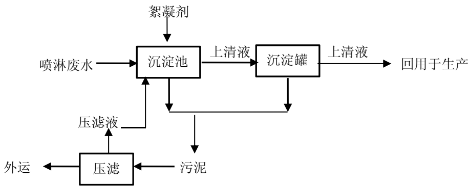
图 7-1 生产废水工艺流程图
