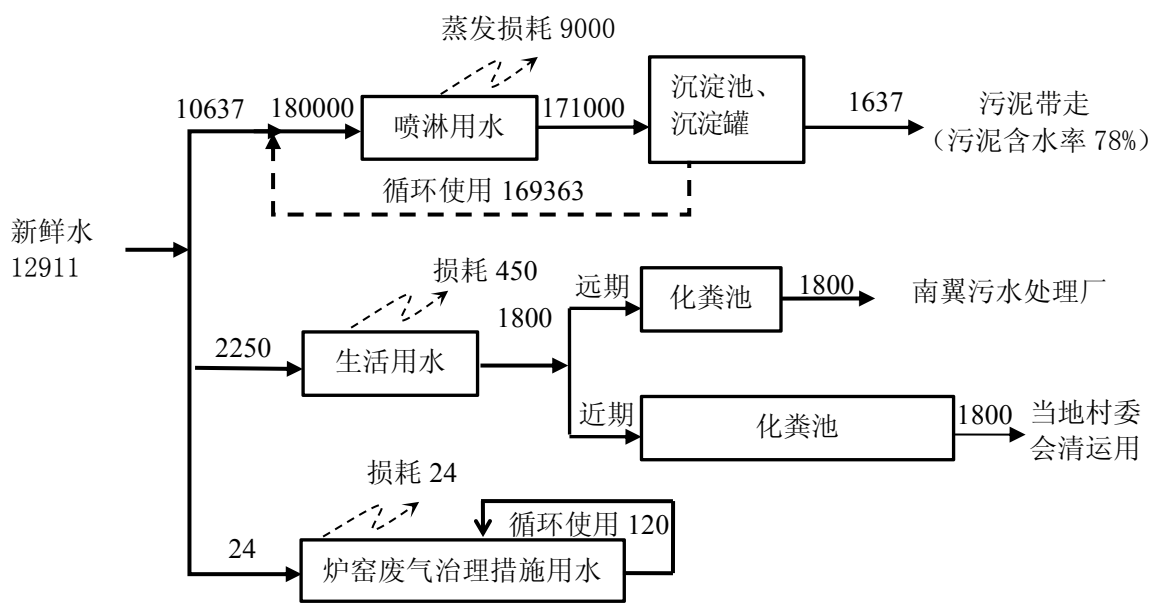
图 3-3 改扩建后项目水平衡图（单位：t/a）
