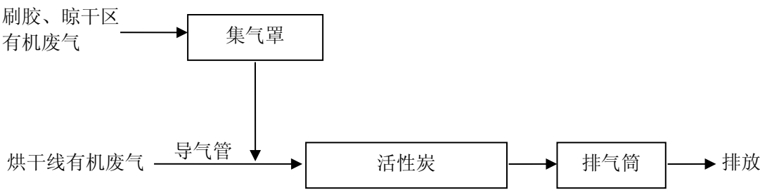
图 7-2 项目有机废气治理措施工艺流程图
