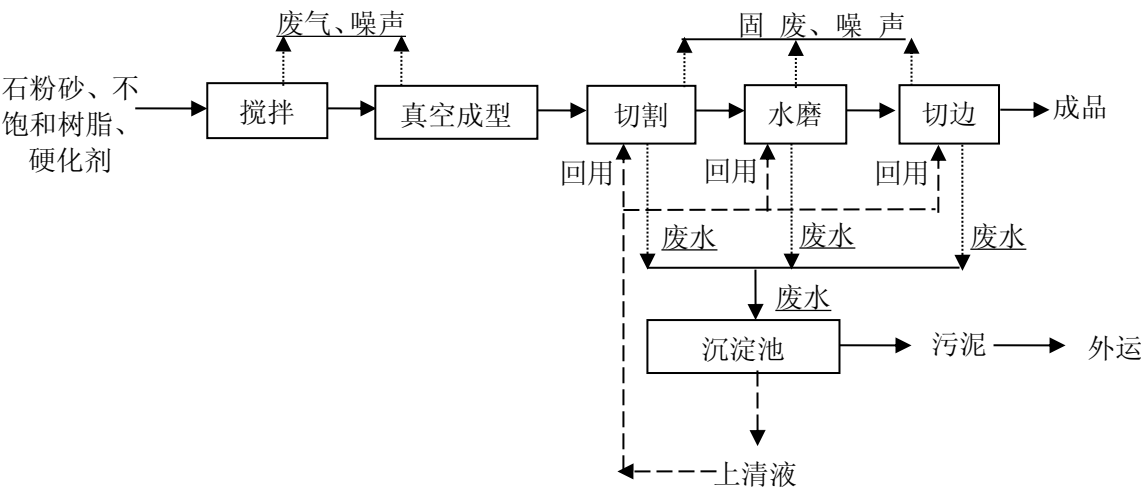
图 3-1 原有项目人造石生产工艺流程图
