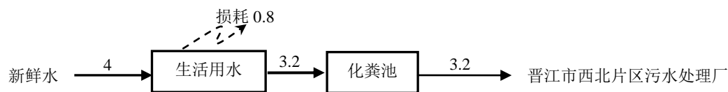
图 2.1 项目水平衡图 单位 m 3 /d
